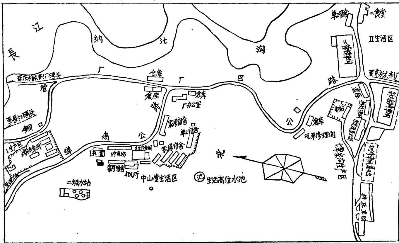
重庆铜管厂厂区平面示意图
