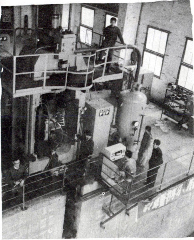
六百吨立式水压机
