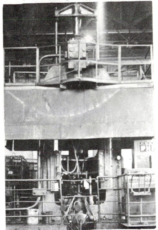
六百吨立式水压机正面照
