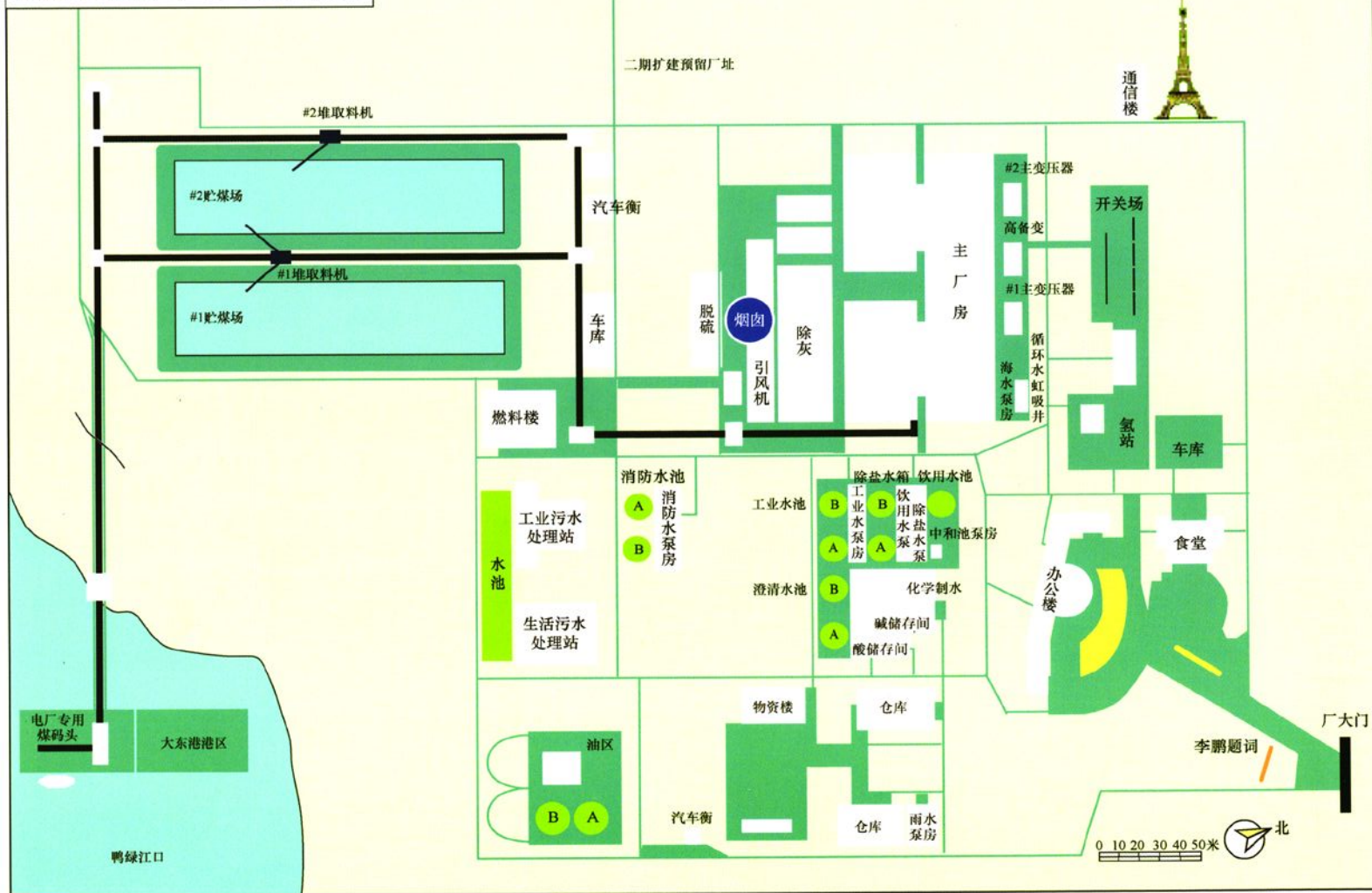
华能丹东电厂厂区平面示意图
