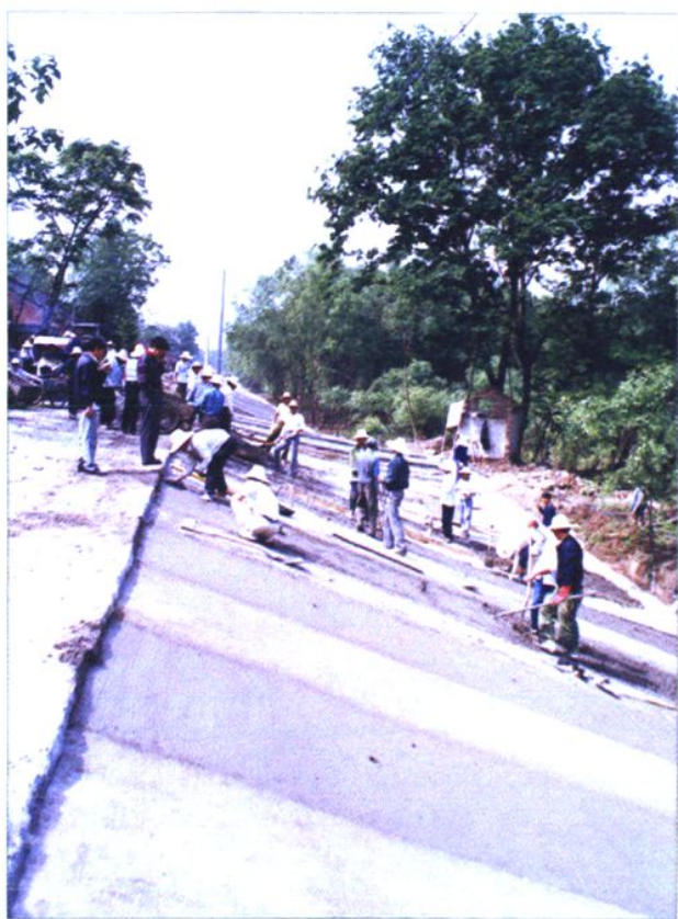
长江主江堤护坡工程
