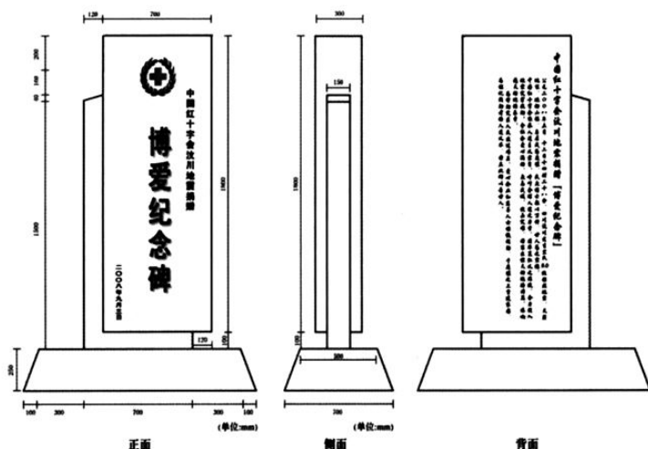
纪念碑平面图
