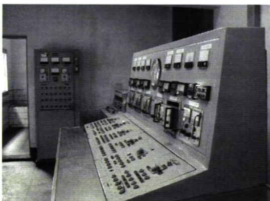
粉碎机自动控制室
