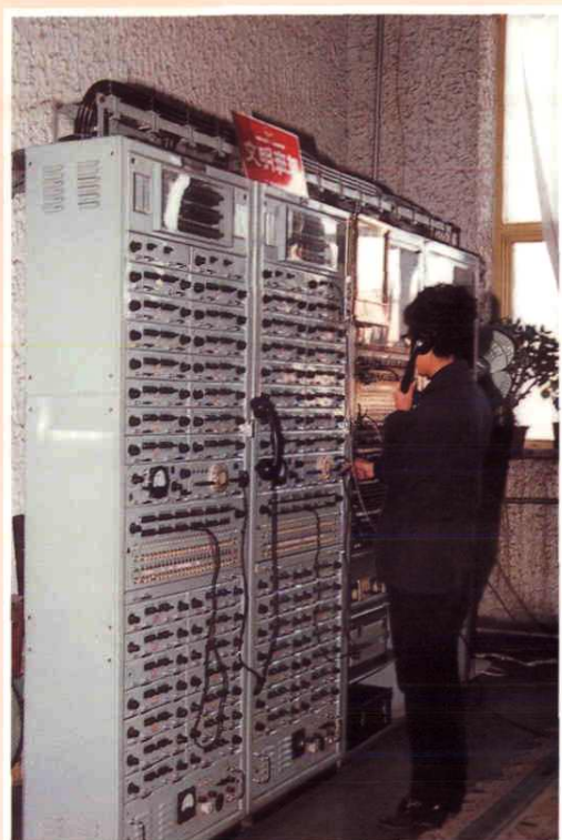
会议电话机房(1990年摄)
