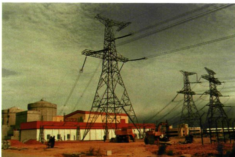
500\text{kV} 广东大亚湾核(电站)—增(城)输电线路工程(1992)
