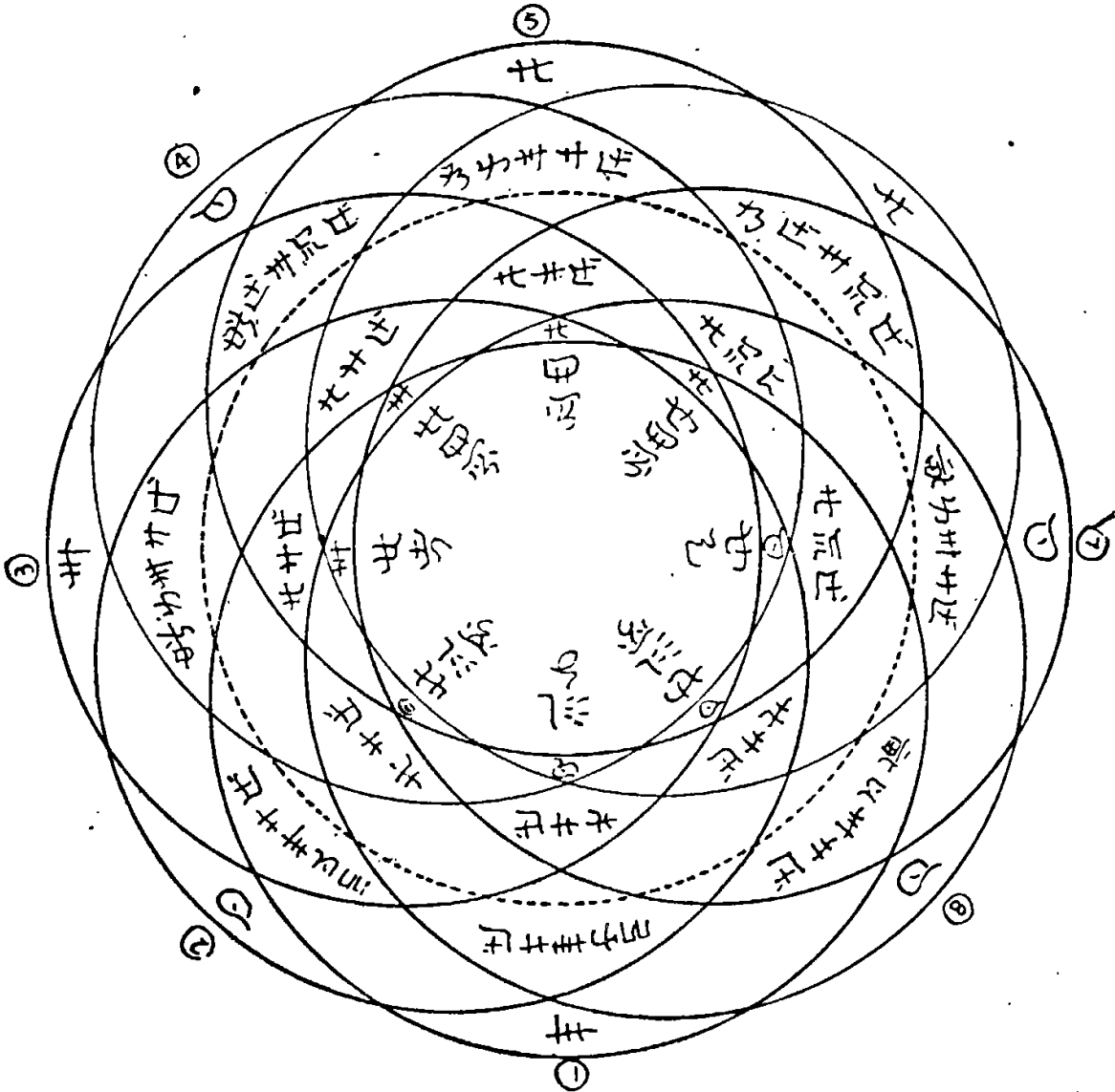
清浊二气运行的轨道图
