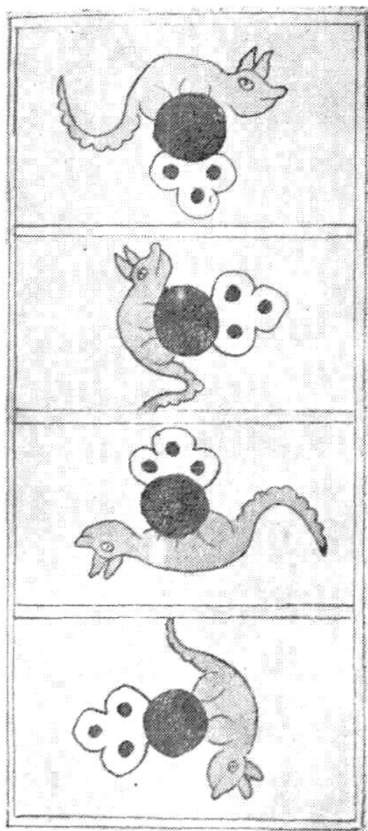
图10·2 耳苏人『母虎历书』封底四幅虎踩天球图。此图采自四川甘洛县寨平公社腊摩歹（母虎村）西番耳苏人巫师杨光银珍藏的『母虎历书』。上图为原件照片。下图为复制件。天球上所附三星表示众星。
