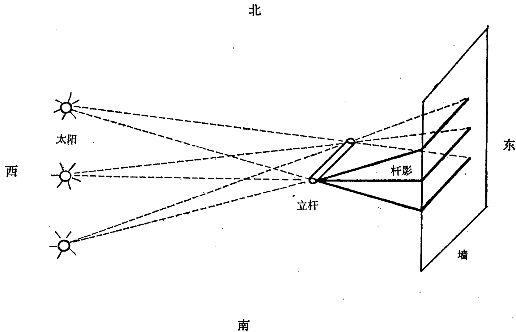
图4.4 阿克甲兹利用日落时投在西墙上的杆影定季节的方法
