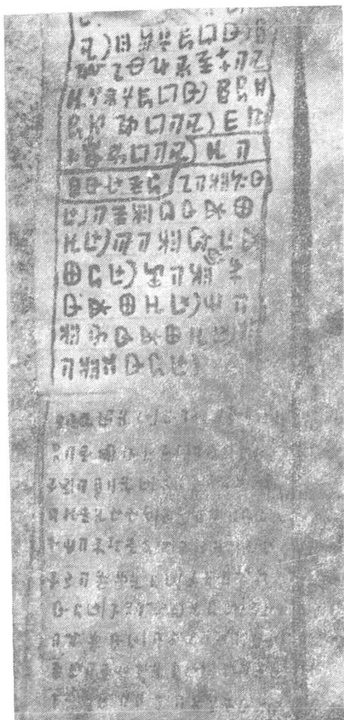
图3.6 《日算书》中有关恒星知识的一页
