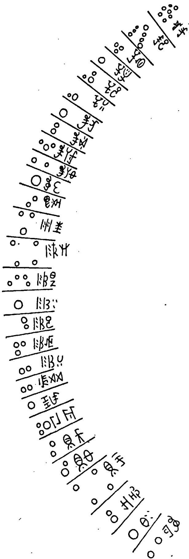
图 3·8 沙正才的二十八宿星图
