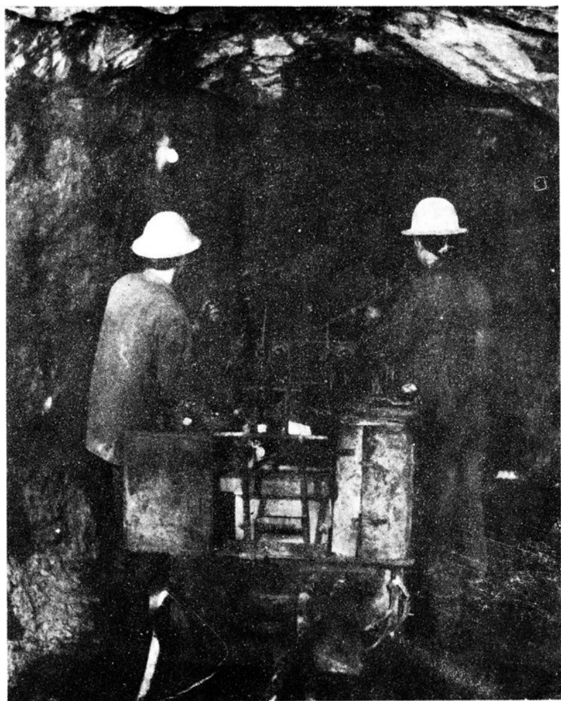
左：横山岭工区的 矿工们在使用 凿岩台车掘进 平巷
