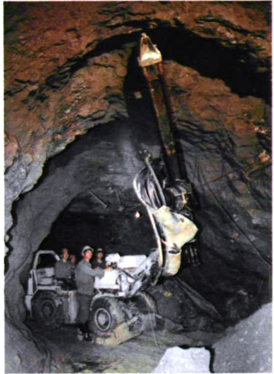
鑿岩臺車
