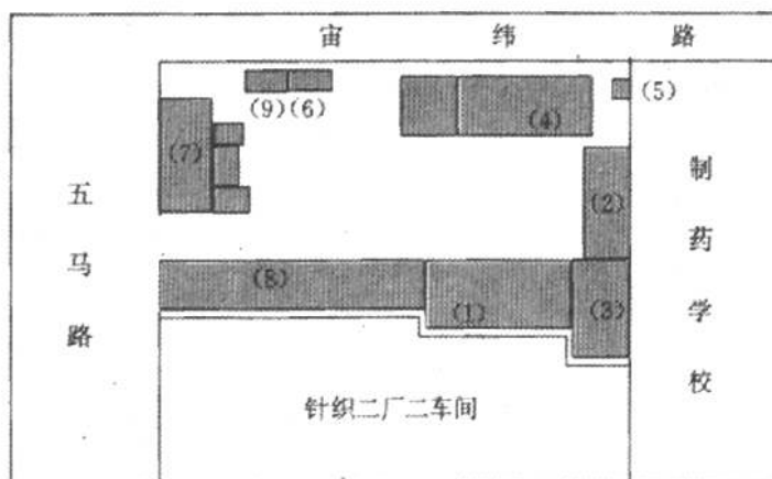
宙纬路实验药厂总平面图
