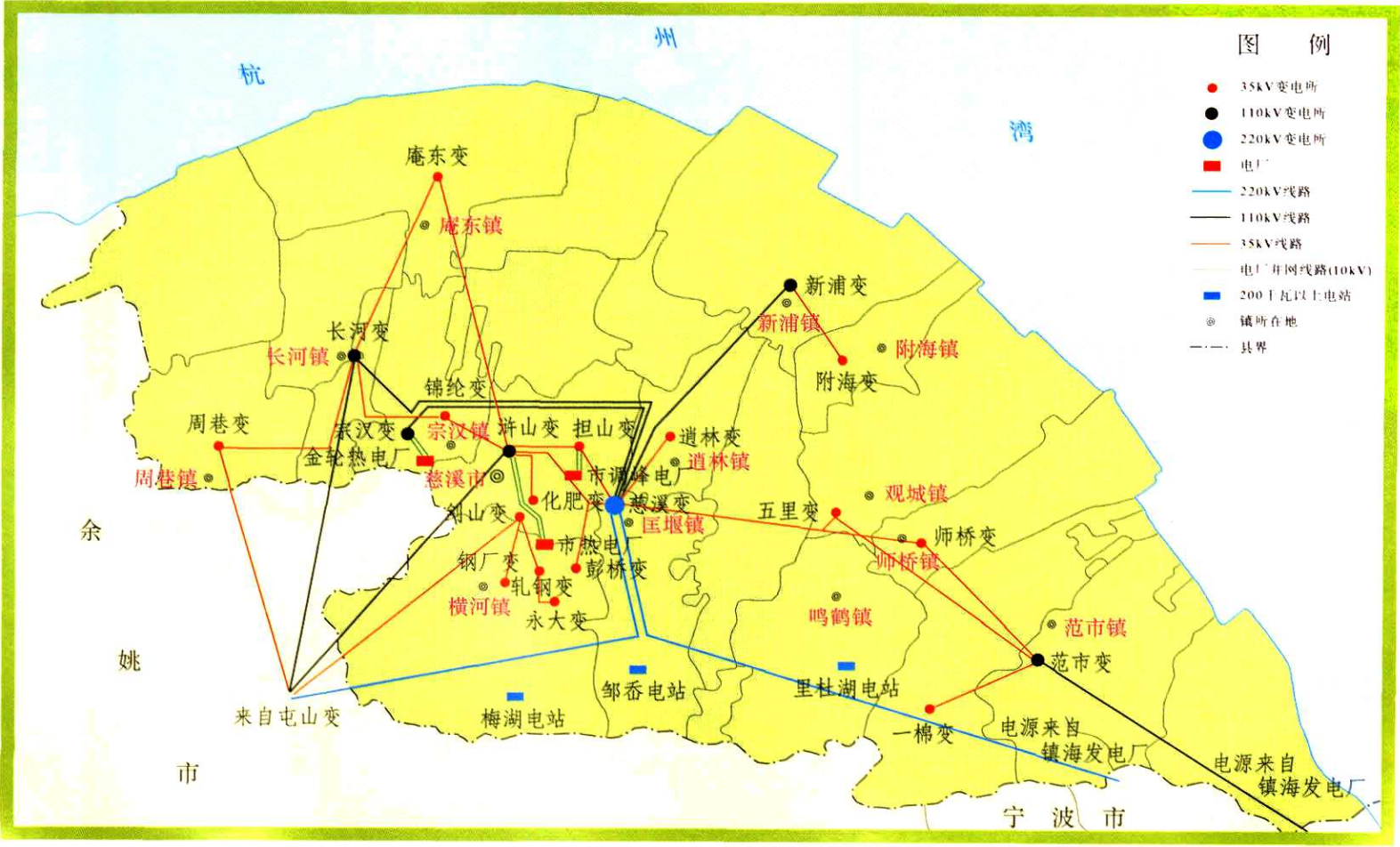
慈溪市35千伏及以上电网地理接线示意图 ( 1995 年 )
