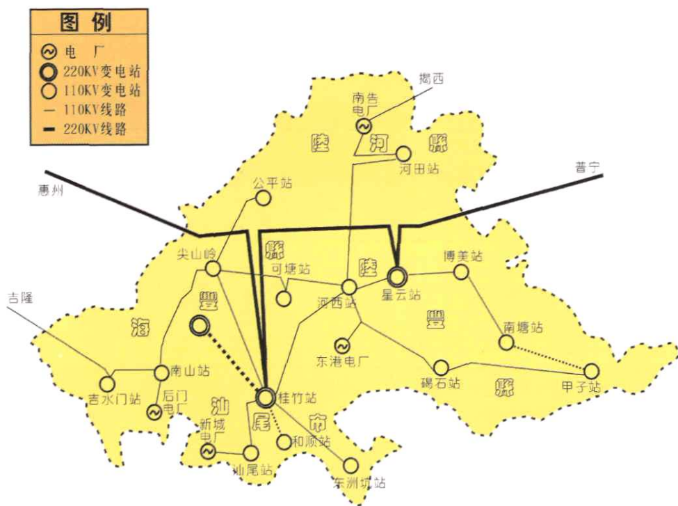
汕尾电网地理结线示意图
