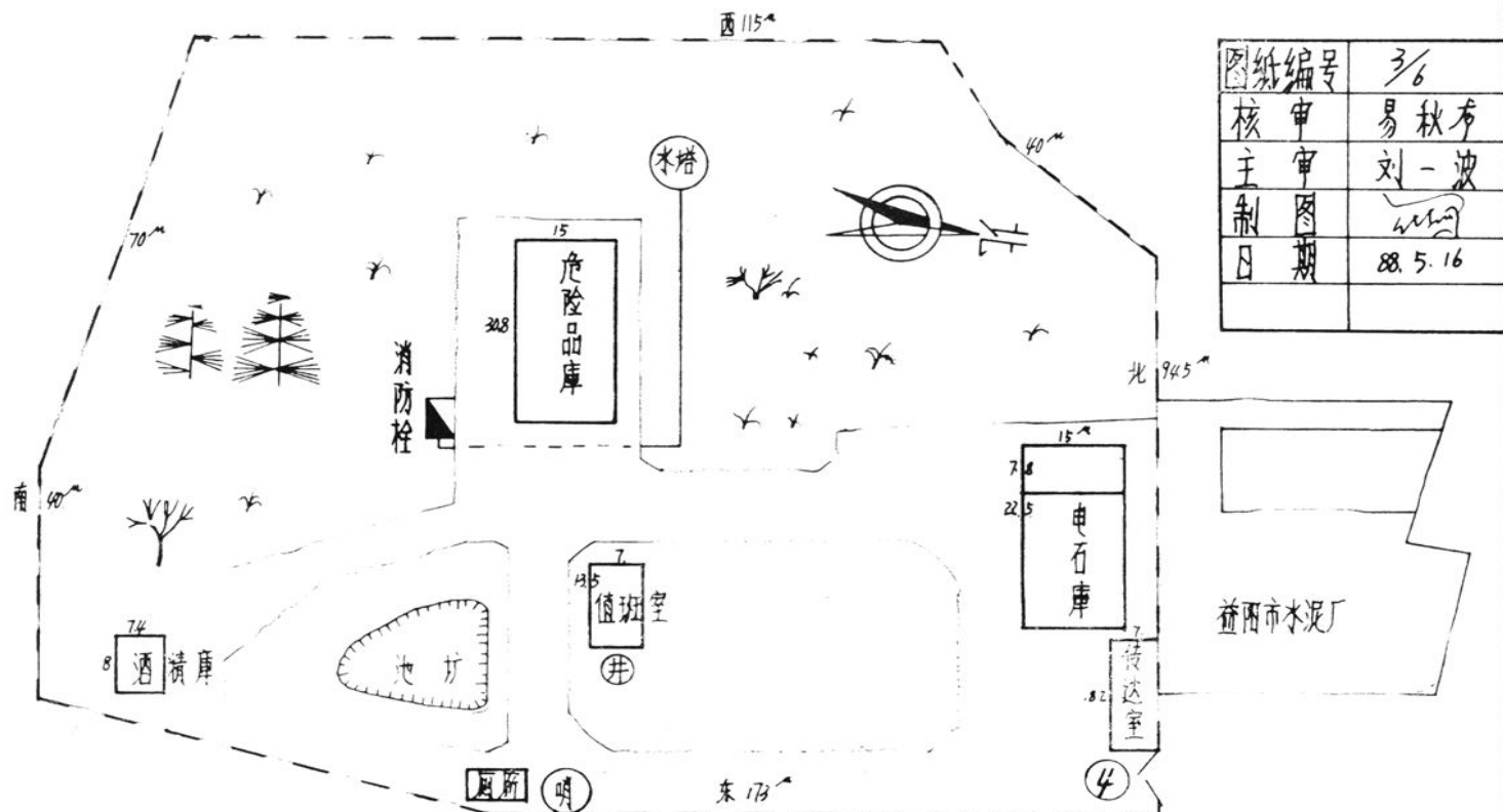
④ 益阳地区轻化建材公司第一仓库(危险品库)平面图 1:1000
