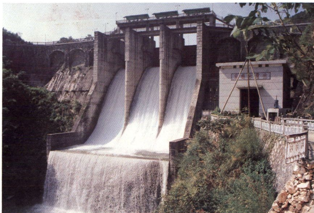
返步桥水库大坝全景
