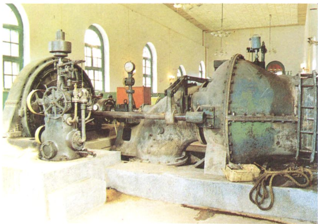
原石龙坝电站240K W 水轮发电机
