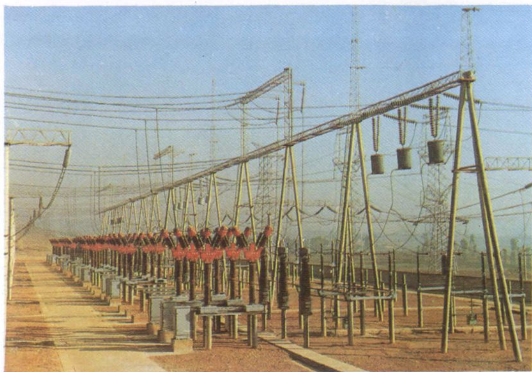
220 K V 东郊变电站开关场
