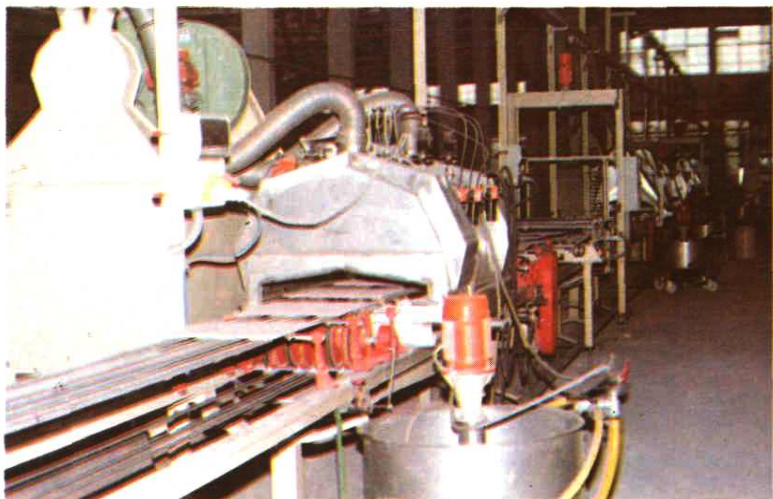
自贡市建陶总厂 引进年产 150 万 m^2 瓷质砖生产线
