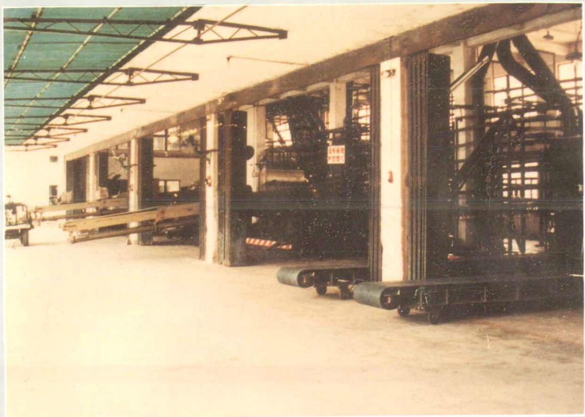
广州邮政枢纽总进口车间 1982 年建成投产。图为接收邮件的带式输送机群。
