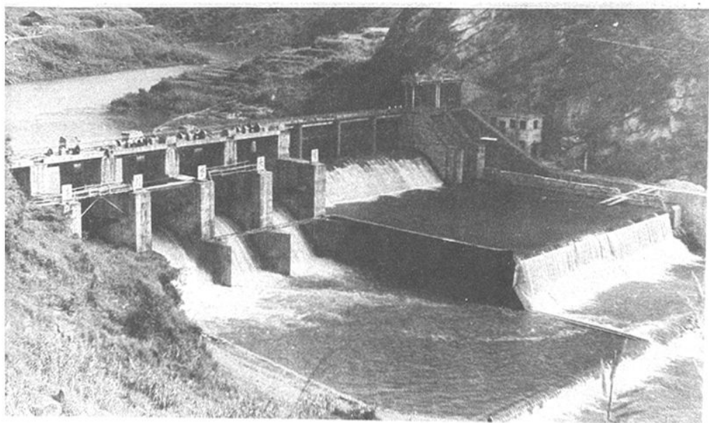
玉溪河引水工程进水口
