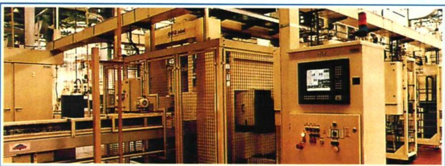
缸盖变余量铣削机床(发动机)
