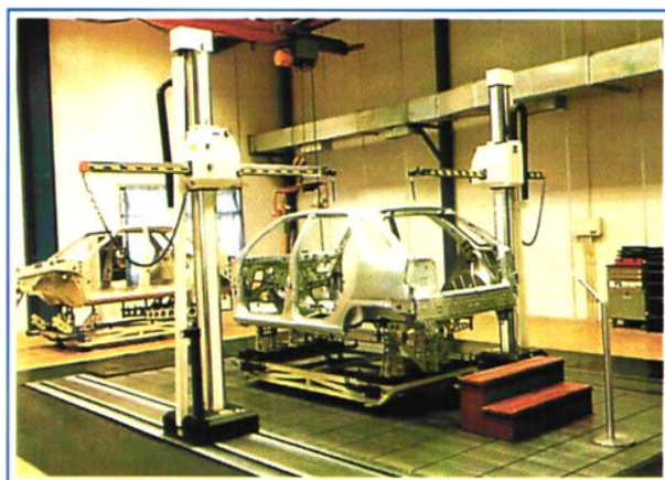
三坐标测量仪
