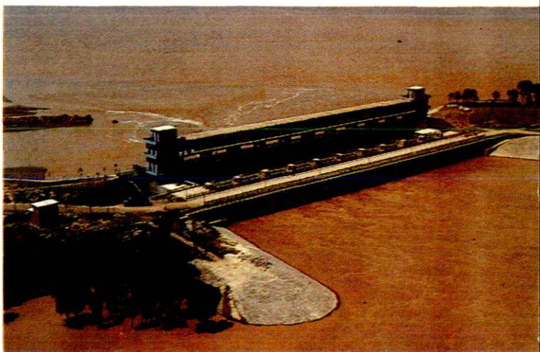
1982年8月黄河大洪水时，东平湖滞洪水库十里堡进湖闸启闸分洪 (殷鹤仙摄)
