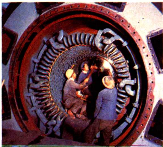
发电机定子检修
