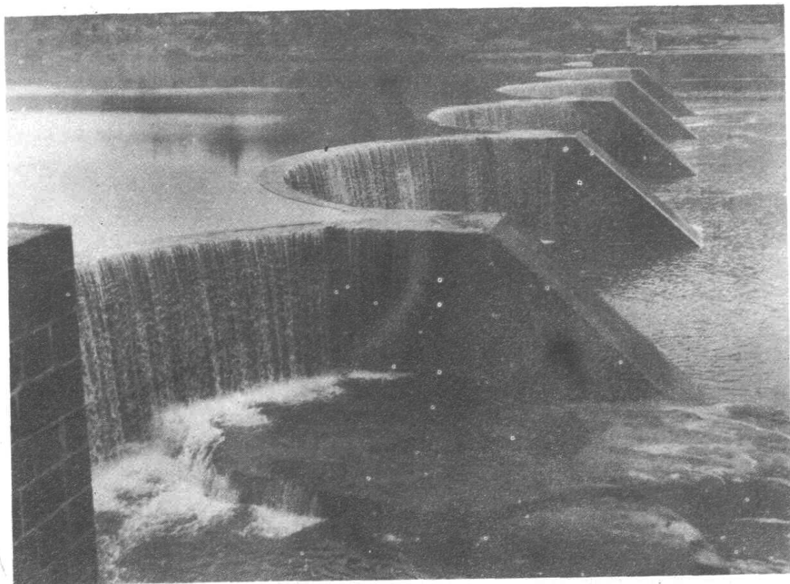
漏水垭水电站拦河坝
