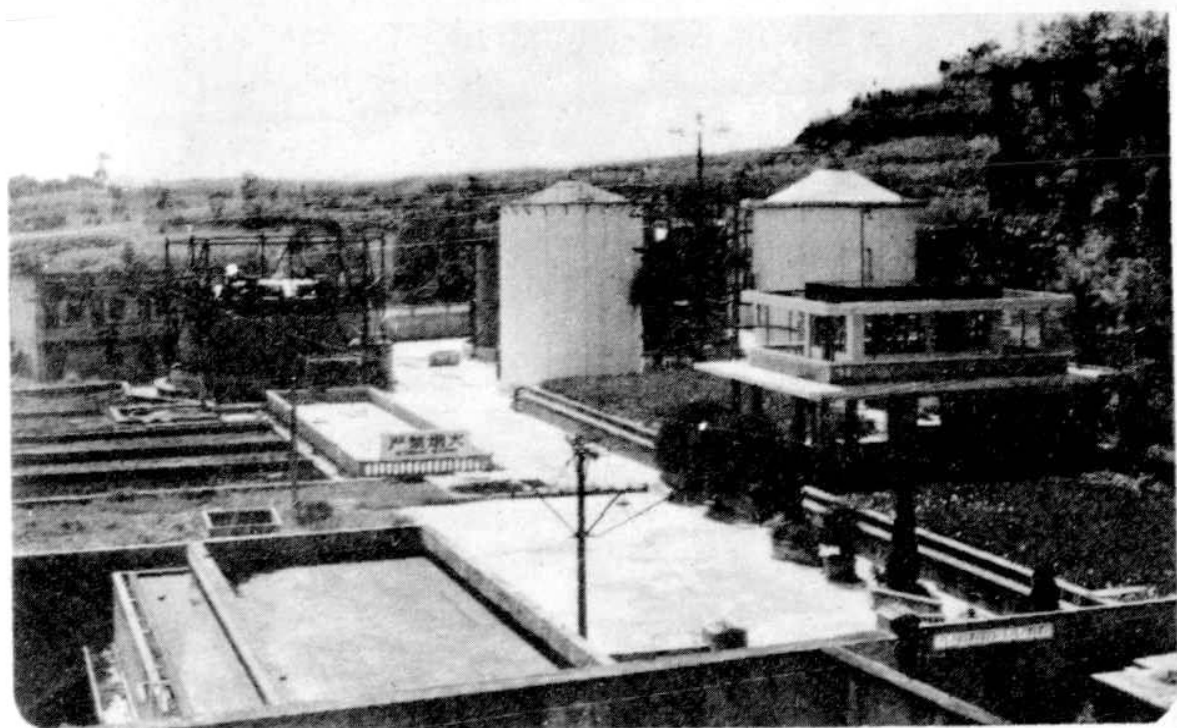
乐至县酒厂沼气集中供气工程鸟瞰 (1989)
