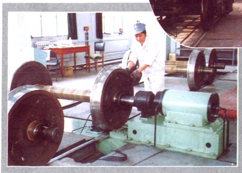
轴承 压装
