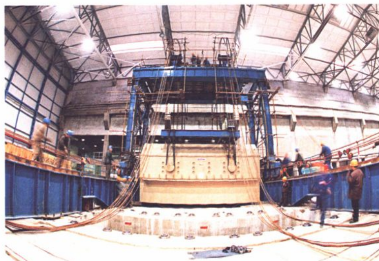
2002年12月，石家庄热电厂技改工程22号汽轮机安装现场
