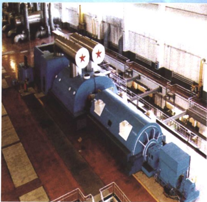
由河北电建二公司承建的邯郸热电厂技改工程20万千瓦发电机组
