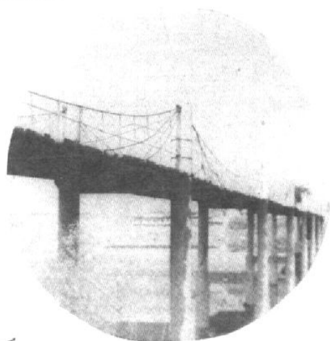
卫河娘娘庙索桥
