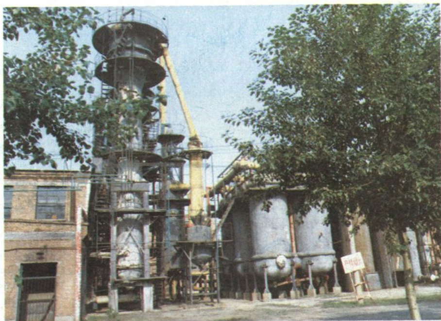
▲ 炼油分厂粗酞氧化炉
