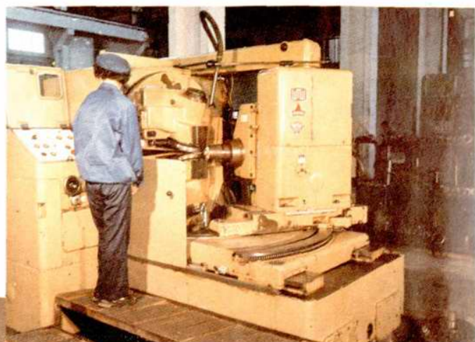
△ 铲齿机床
