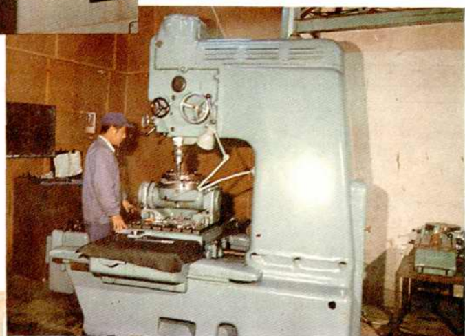
△ 坐标镗床
