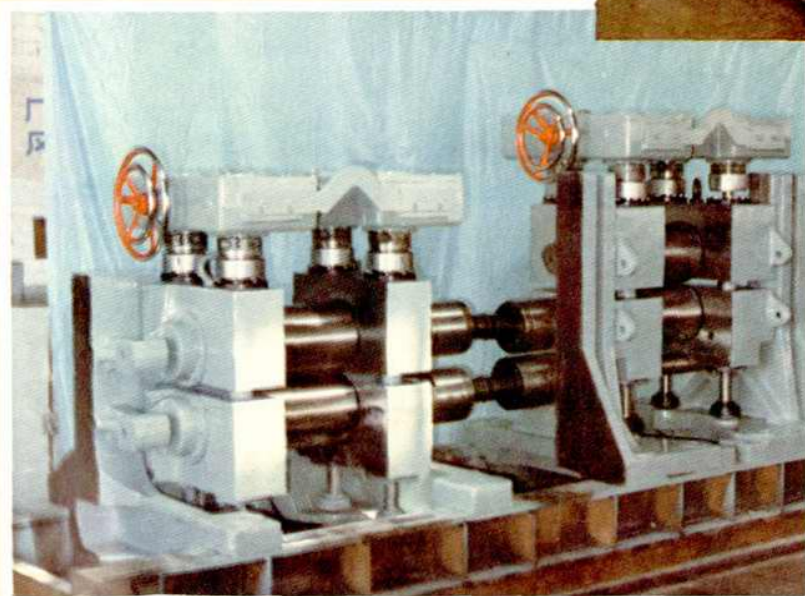
△ 短应力线轧机
