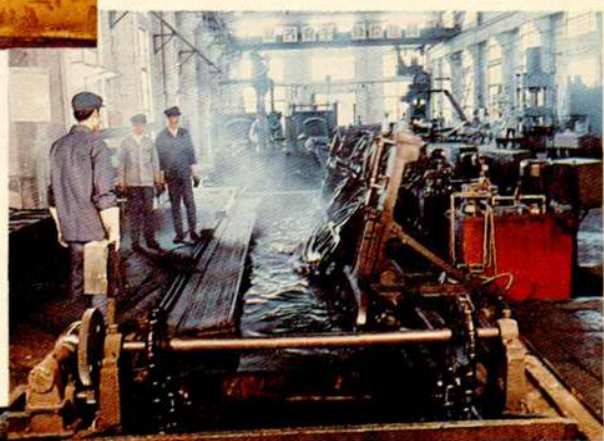
▽ 钢板弹簧淬火
