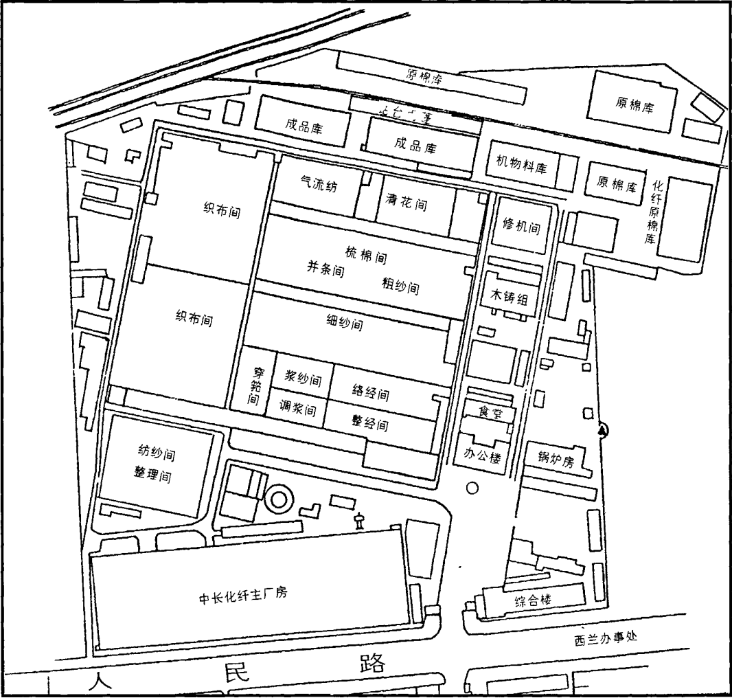
西北二棉集团有限公司生产区平面图
