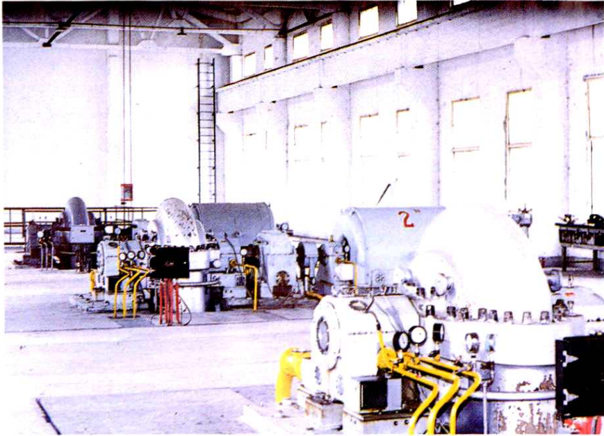
300m 3 /n透平式空压机房。
