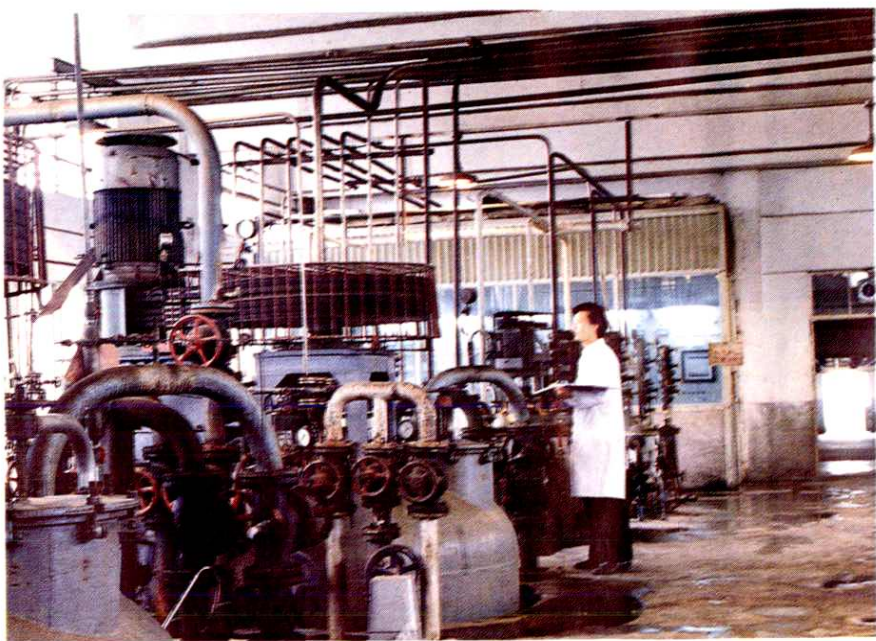
乙酰螺旋霉素车间发酵工场。
