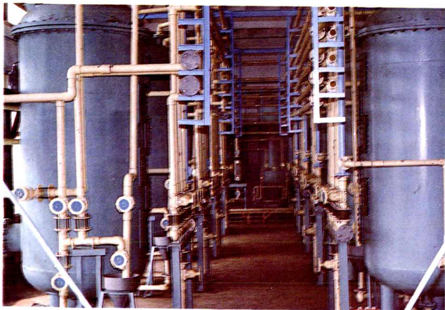
新安装采用ABS管的土霉素车间提炼结晶工场。
