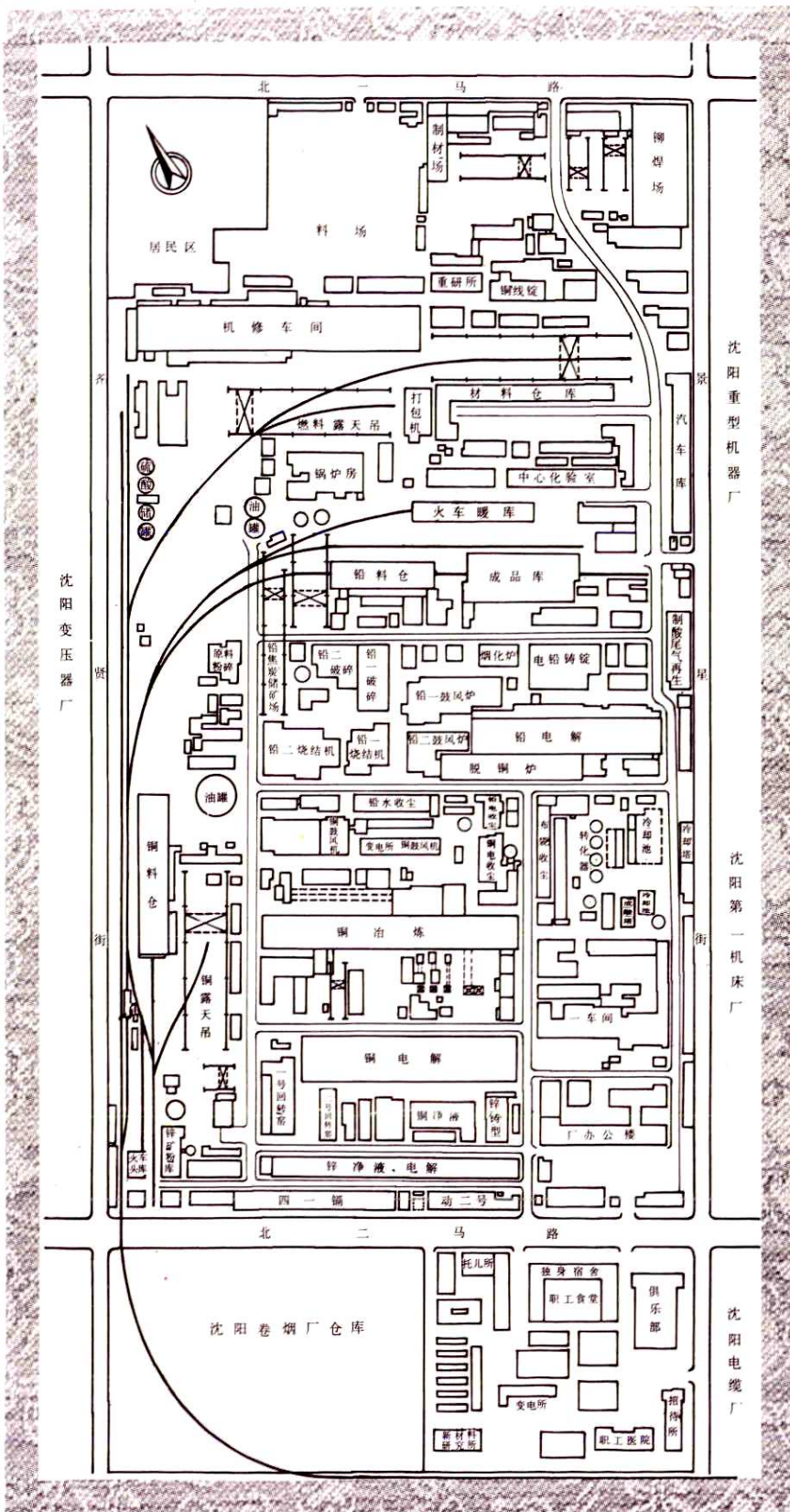
沈阳冶炼厂厂区平面图
