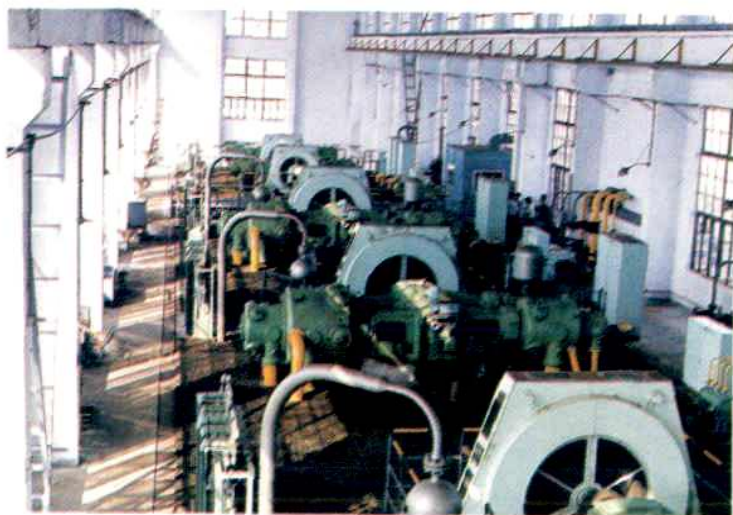
▲ 绵阳南光化工总厂天然气压缩机组。
