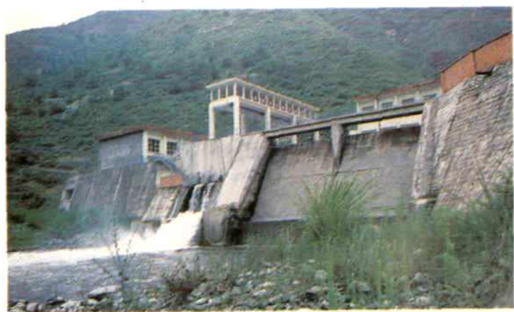
◀平武县电力公司是“省级先进企业”。图为该公司南坝水电厂3 × 1600kw发电站。
