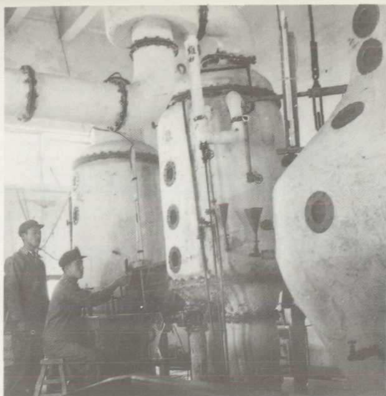
小新滩试验场氯化钾车间
