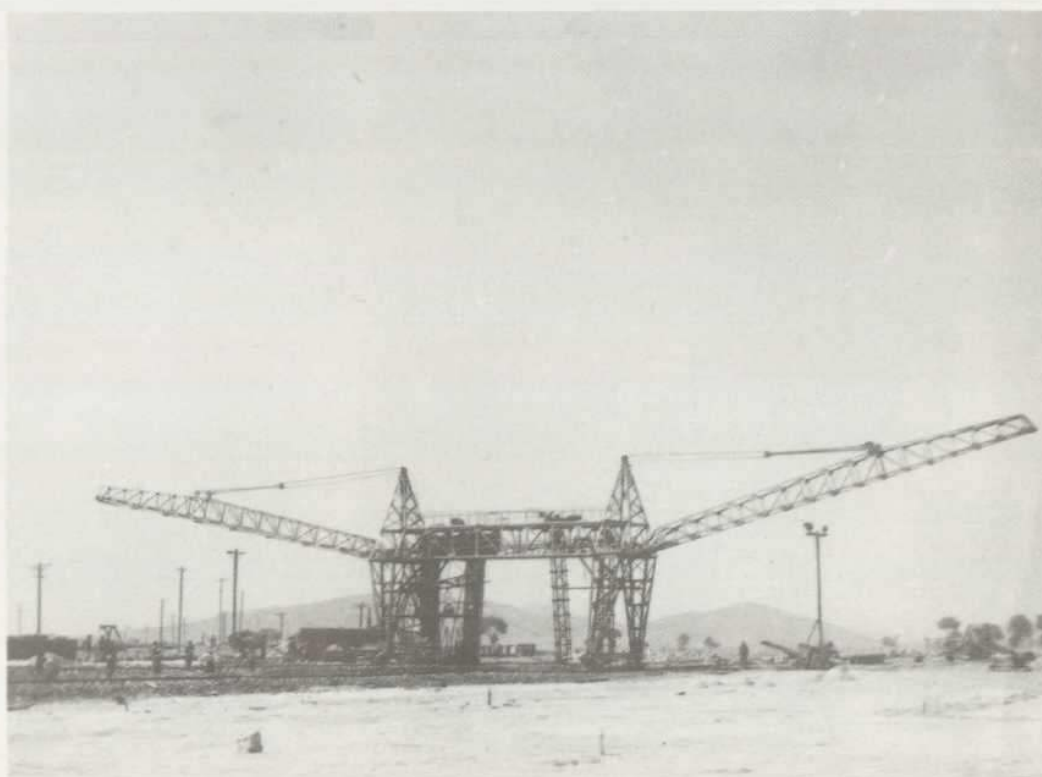
小新滩试验场氯化钾车间
