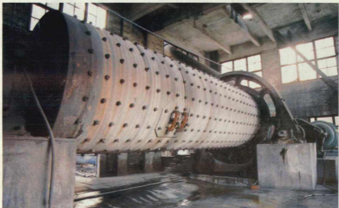
乡镇企业水泥厂 10 万吨水泥生产线
