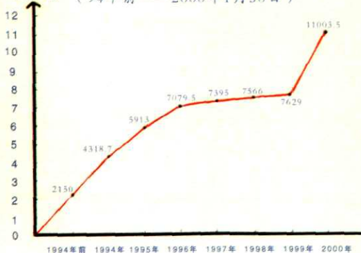
化燃公司氮肥厂碳酸氢铵逐年最高月产量统计图
