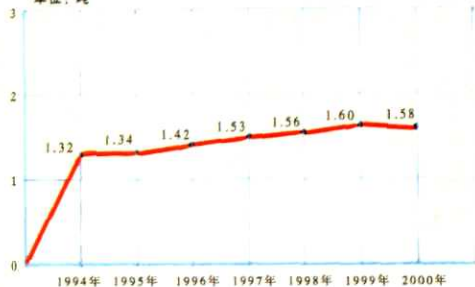
化燃公司氮肥厂碳酸氢铵逐年最高台时产量统计图 (1994年—2000年1月30日)
