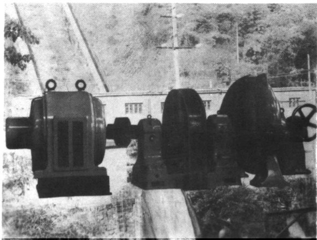
玉溪水电设备厂生产的HL110 - WJ - 50型混流式水轮机组
