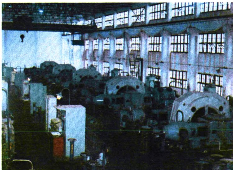
▲ 公司为沾益化肥厂安装的合成氨压缩机组。
