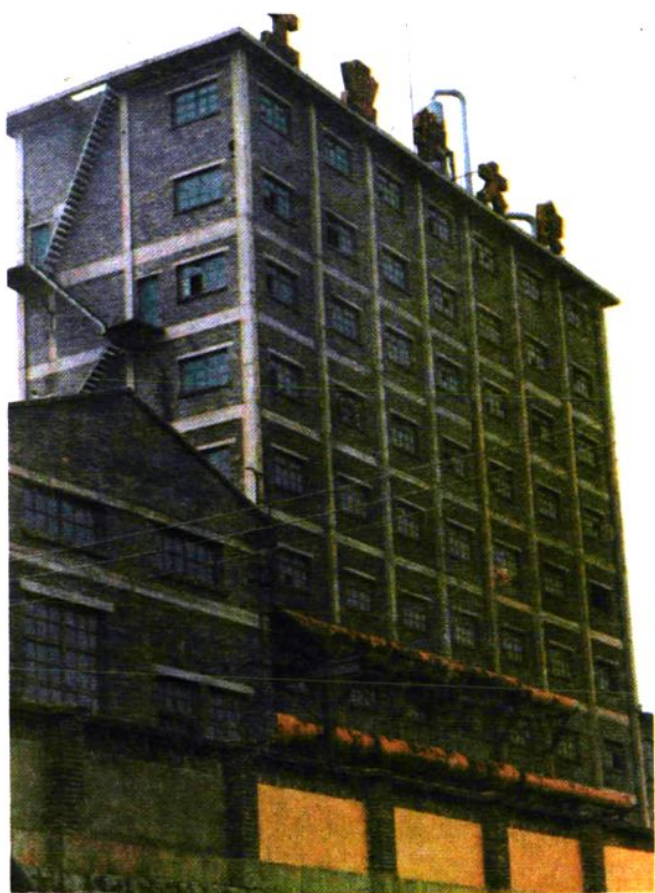
► 公司七十年代初承建的两项 高效多管生产重水（氘）的军工 项目之一——云南氮肥厂748工程。 图为748工程氨精馏主厂房。
