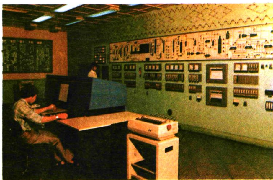
▼ 公司安装的云南天然气化工厂合成氨装置的主控室。
