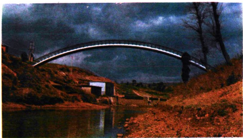
◀ 公司施工的云南磷肥厂供水系统工程之一——“管拱桥”。整体是跨距62米，自重25吨的双管新型管道跨越结构，为云南省第一座跨越管道结
