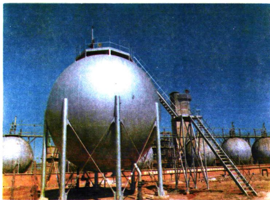
▲ 公司为沾益化肥厂安装组焊的200M 3 、400M 3 球罐群。
