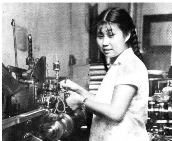
印刷厂职工正在进行化铅和铸字作业
