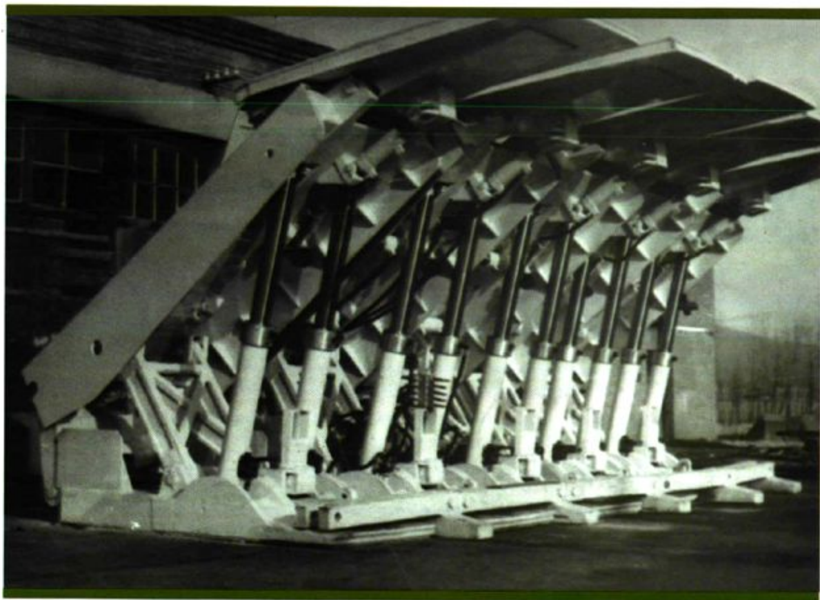
1976年平顶山煤矿机械厂生产的我国第一套掩护式液压支架（ZYZ-1型）
