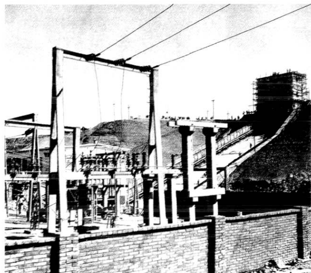
正在建设中的五级电站升压站
