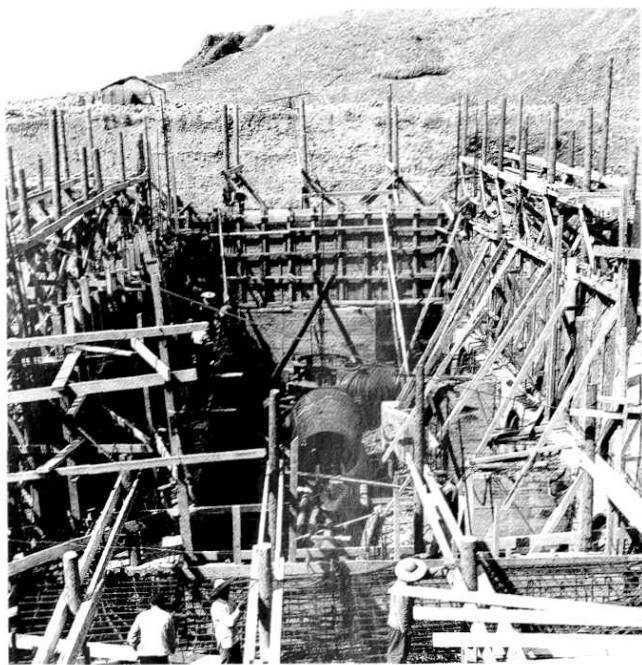
五级电站机坑预埋(1965)
