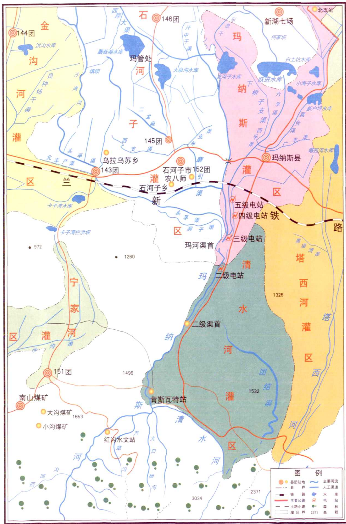
新疆石河子红山嘴水力发电厂四站示意图
