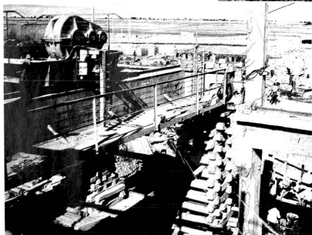
施工中的五级电站土 法上马，采用木枕井字架 安装起重机(1965)
