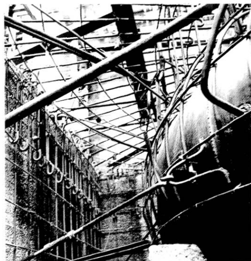
五级电站机组涡壳在预埋中(1965)
