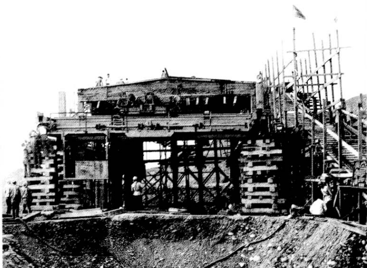
正在修建中的五级电站厂房
