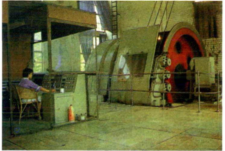
长广煤矿公司七矿落地多绳绞车房
