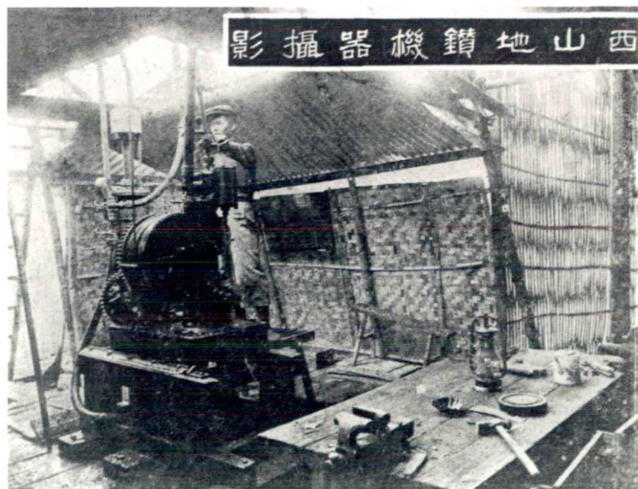
1920年长兴煤矿的钻机在西山井田钻探情况
