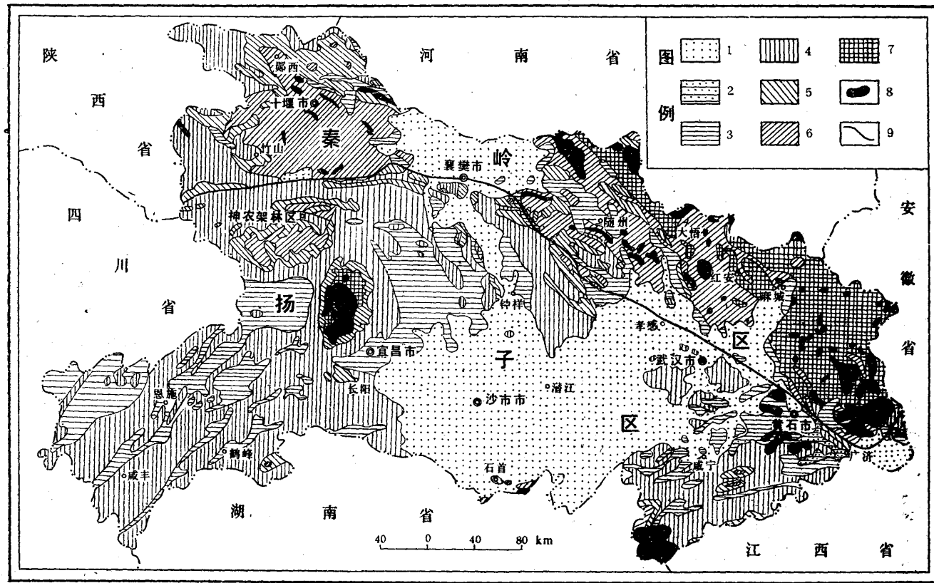
图 I-1 湖北省地层分布略图
