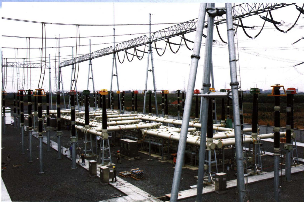
全国首创“两型一化”无人值班变电站建设试点——500 千伏惠泉(锡西南)变电站
