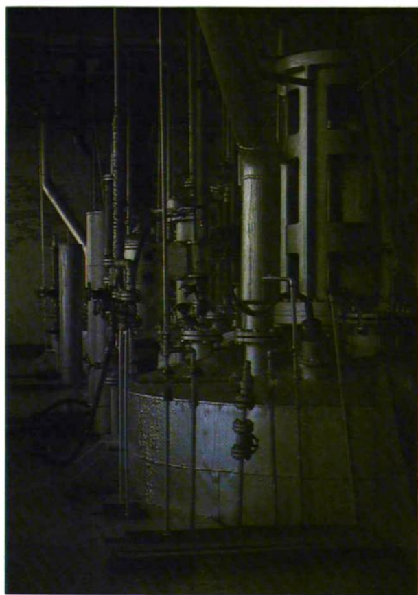
大连油漆厂的醇酸树脂漆生产装置
