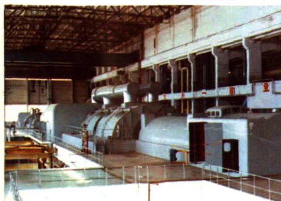
汽轮发电机组
