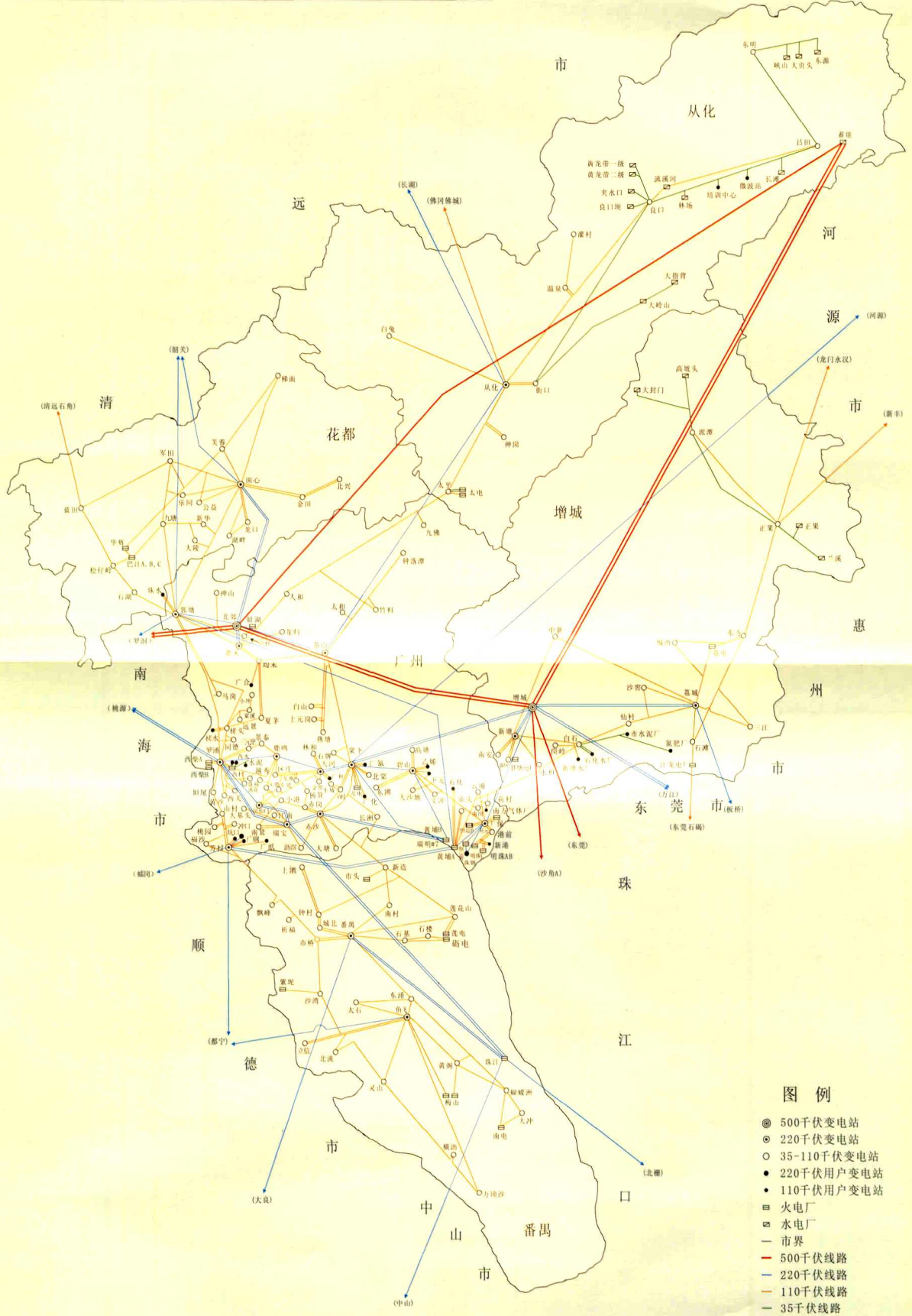
2000年广州地区35—500千伏电网地理接线示意图
