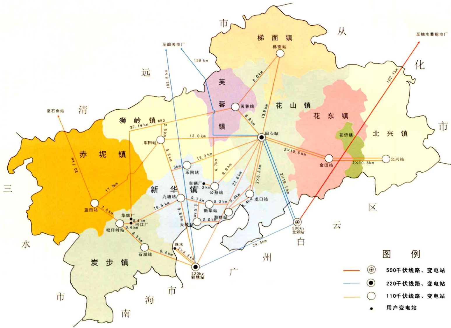
2000年花都110—220千伏电网地理接线示意图
