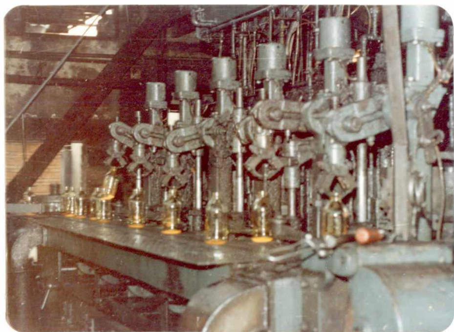
六组单滴料行列式制瓶机
