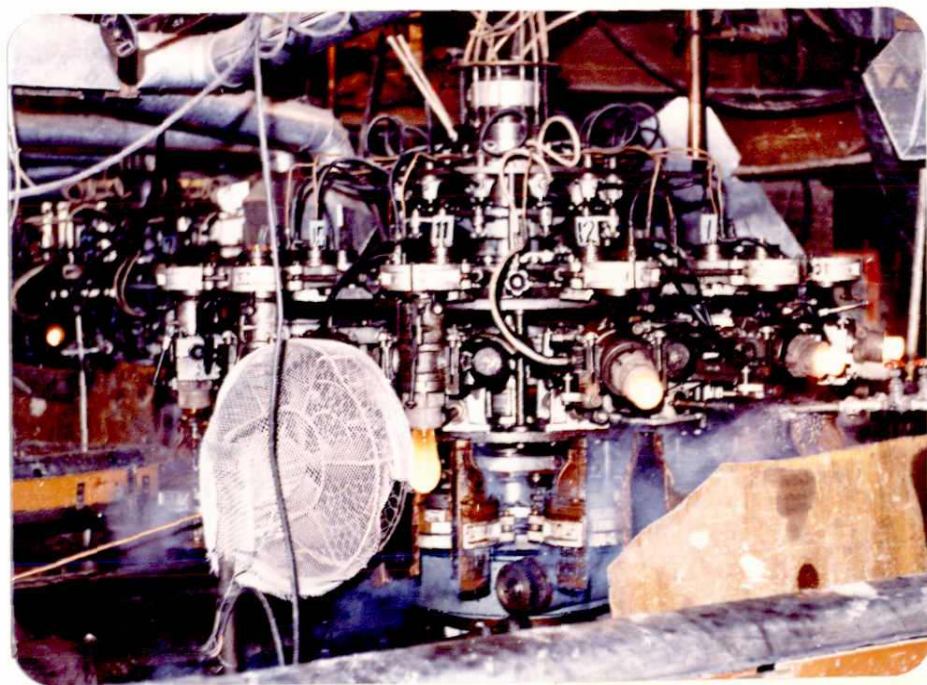
12模自动吹泡机
