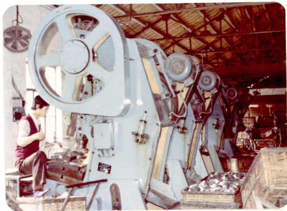
冲床工人在冲压保温瓶外壳
