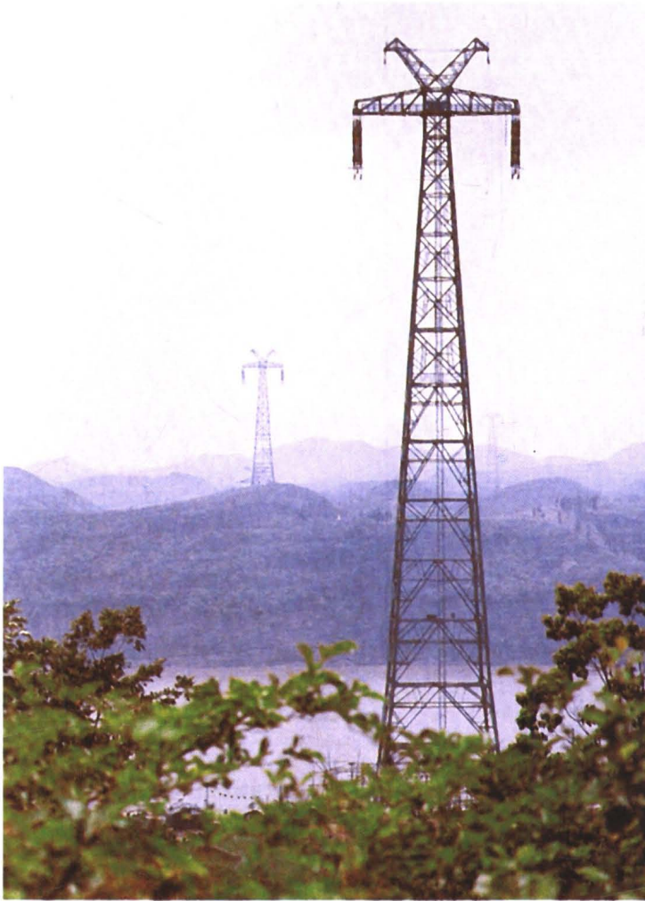
1987年建成的 \pm 500 千伏葛洲坝—上海直流送电线路
