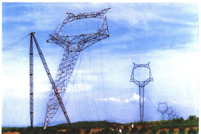
1980年代开发应用拉猫塔整体组立工艺
