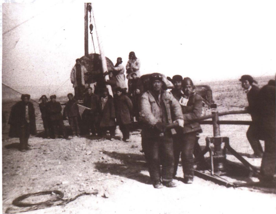
1960年代的送电施工现场，组立杆塔和架线的主要动力器械为人力绞磨
