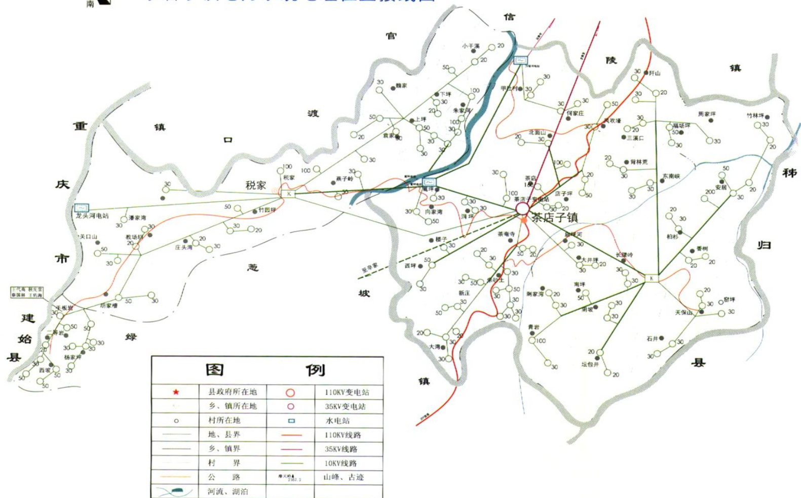
茶店子镇电力系统地理位置接线图
