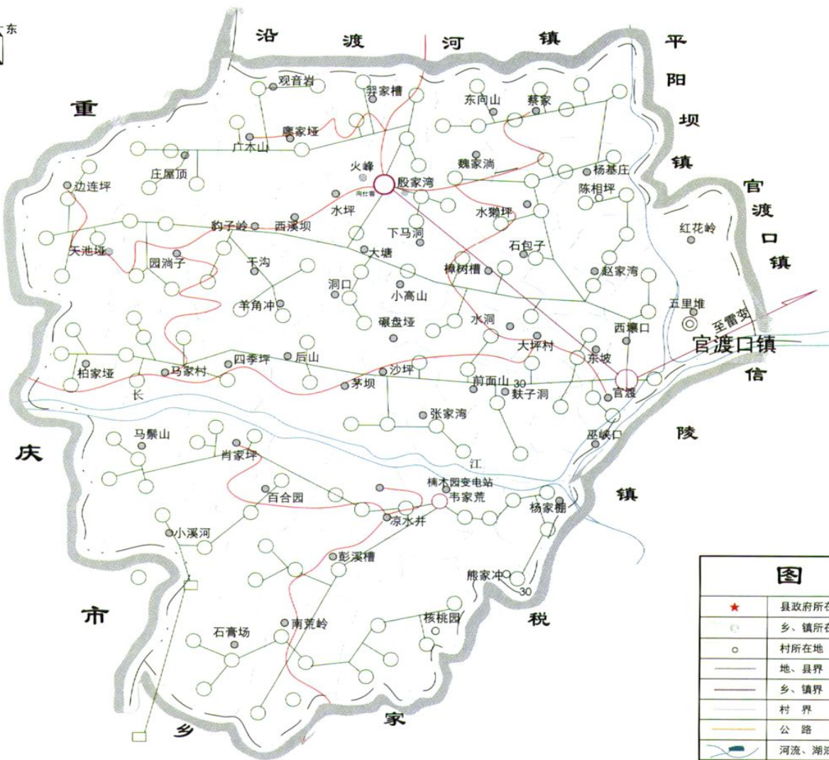
官渡口镇电力系统地理位置接线图
