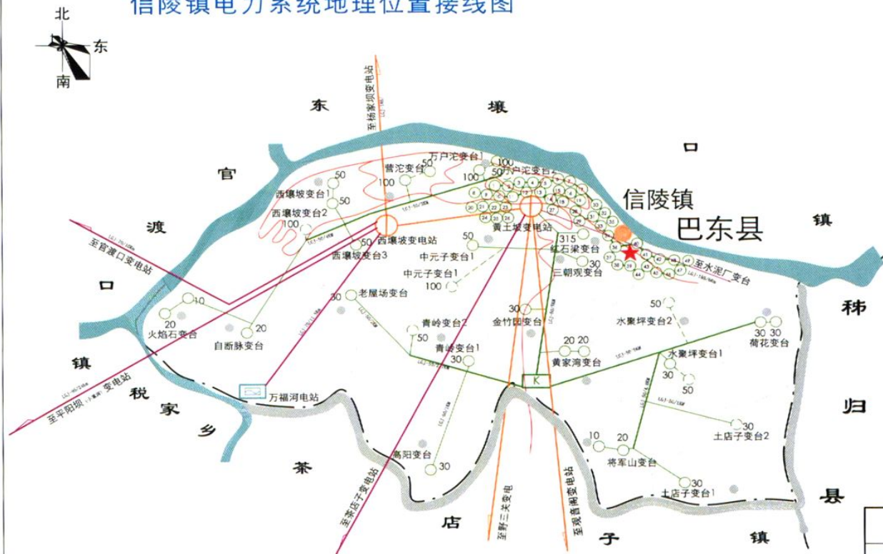
信陵镇电力系统地理位置接线图
