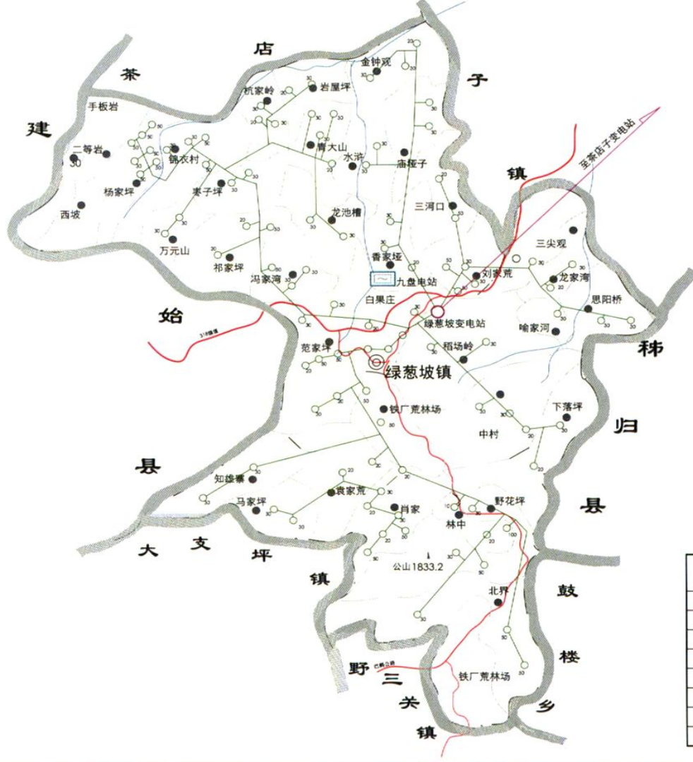
绿葱坡镇电力系统地理位置接线图
